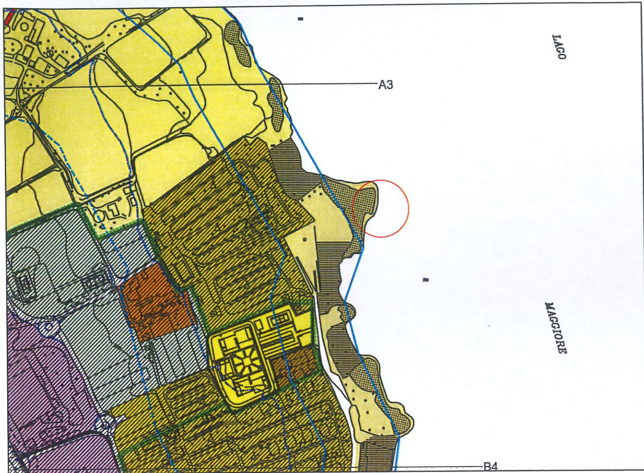
P.R.G.C. comune di Dormelletto - scala 1:5000
