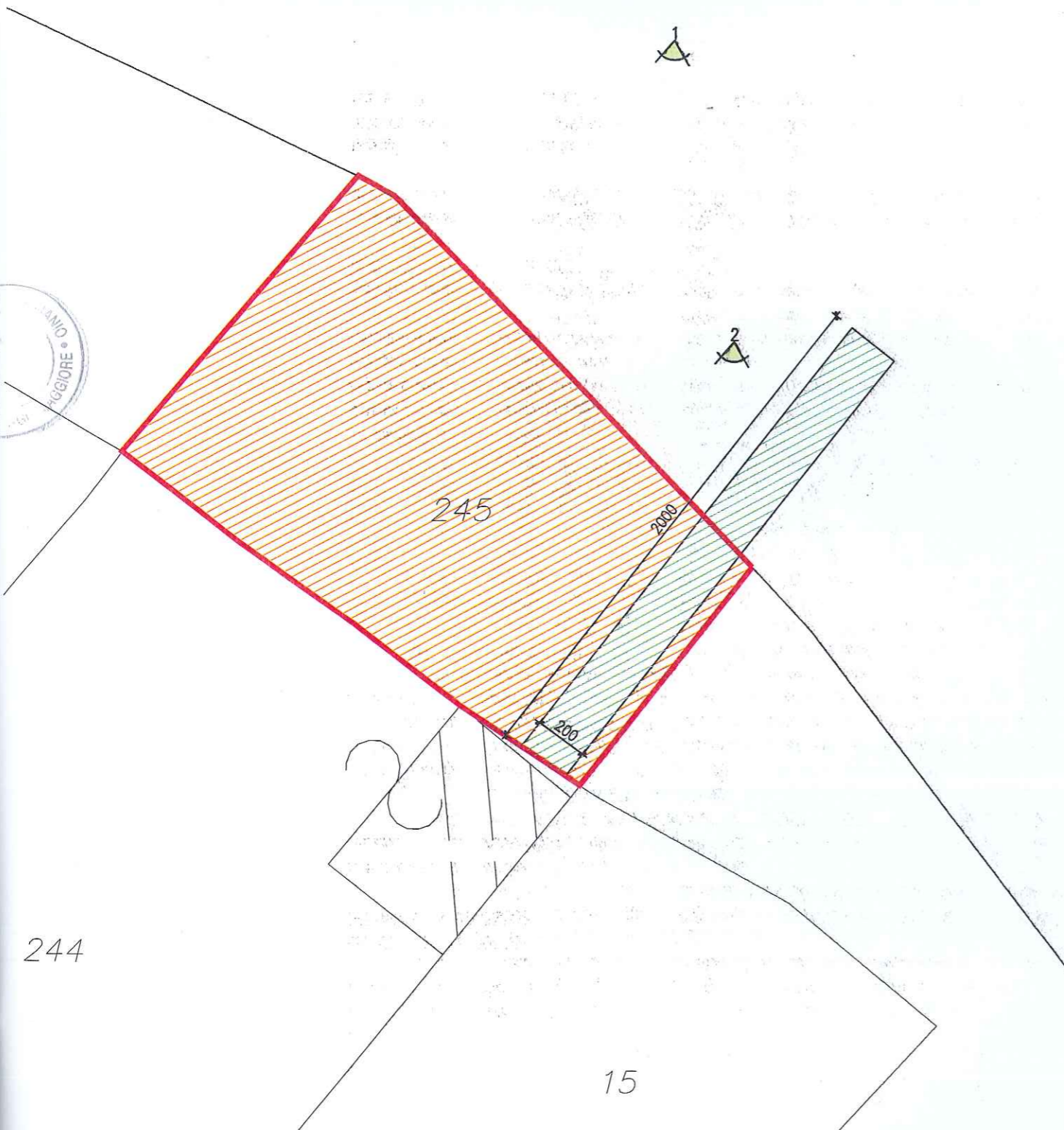
PLANIMETRIA GENERALE - rapp. 1.200
