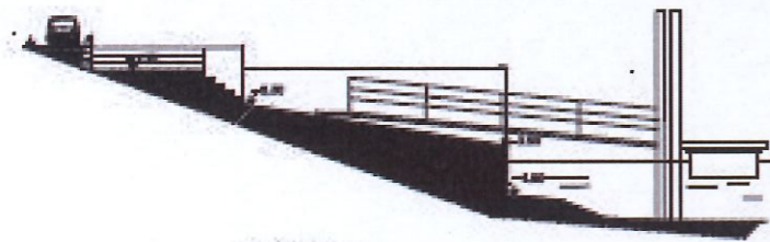
SEZIONE scala 1:100
