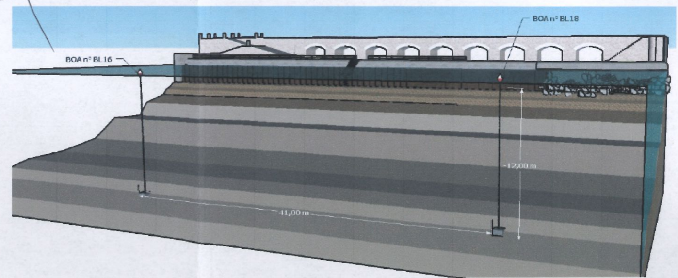
SEZIONE QUOTATA
