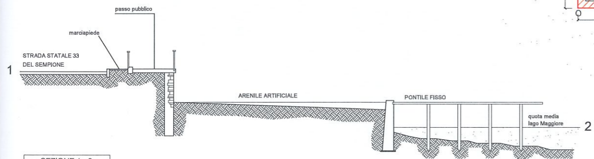
SEZIONE 1 - 2 Scala 1:100
